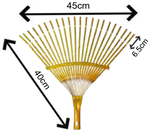
钢铁草耙 (Qty: 36 Pcs X 1 Ctn)
