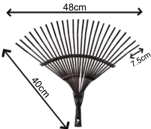
钢铁草耙 (Qty: 30 Pcs X 1 Ctn)
